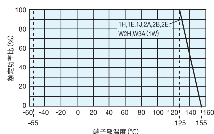
端子部温度
