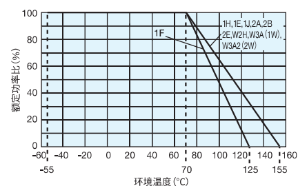
环境温度
